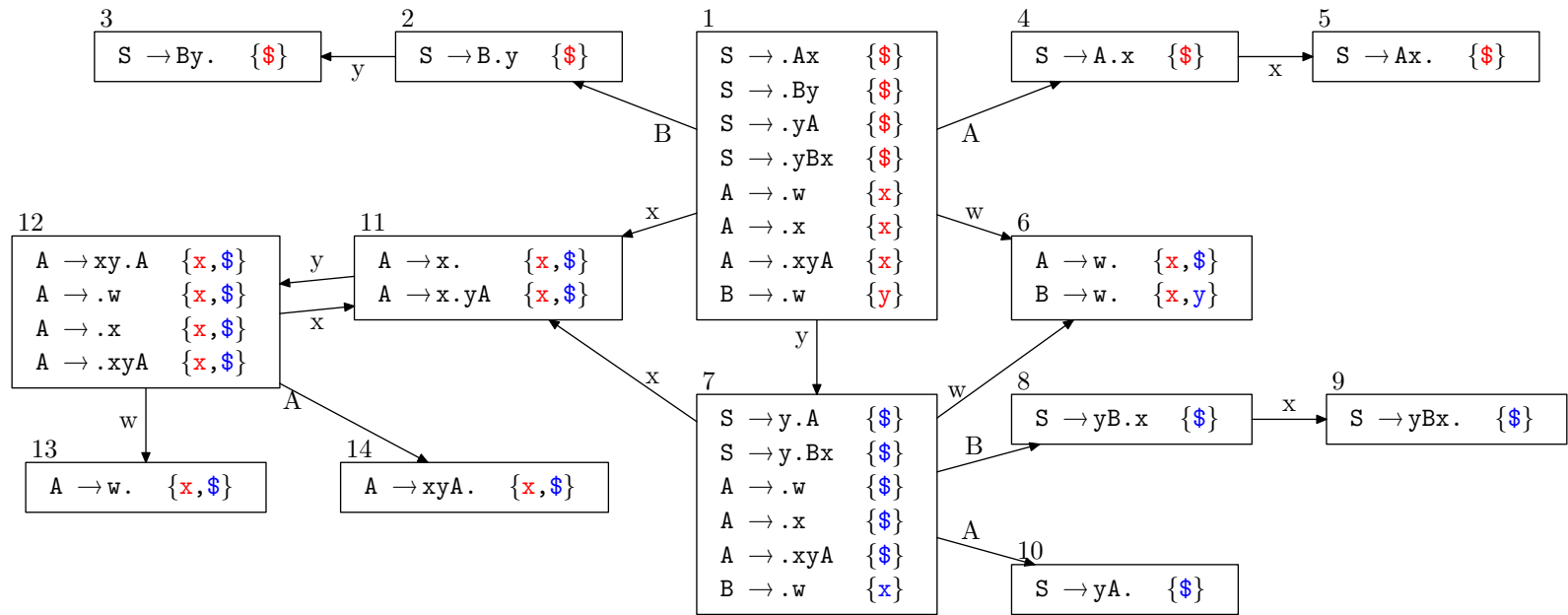
Abbildung 2: LALR(1)-Präfixautomat
