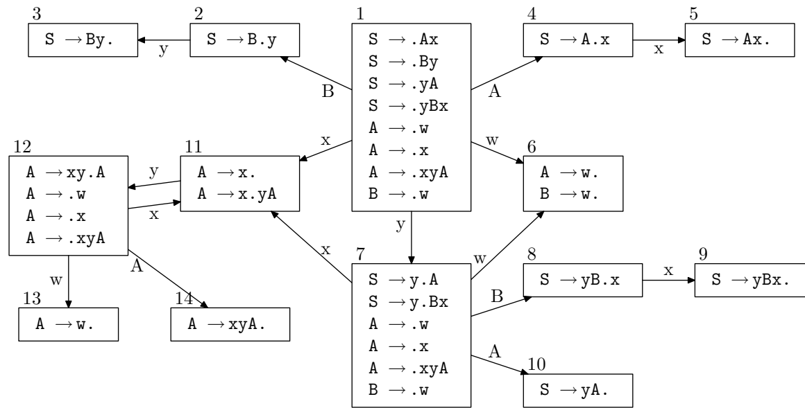
Abbildung 1: LR(0)-Präfixautomat
