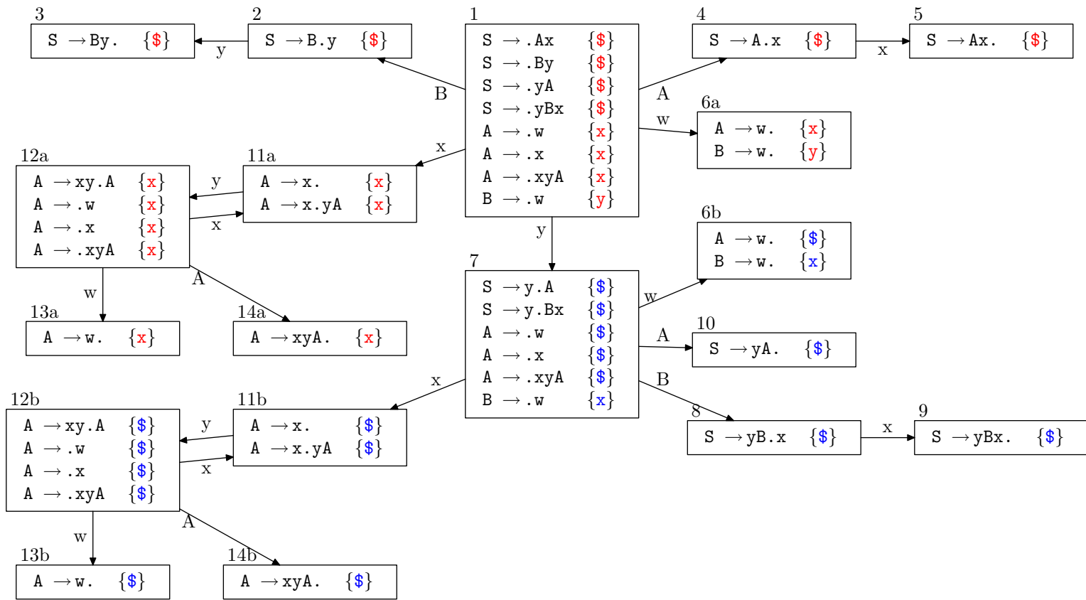
Abbildung 3: LR(1)-Päfixautomat
